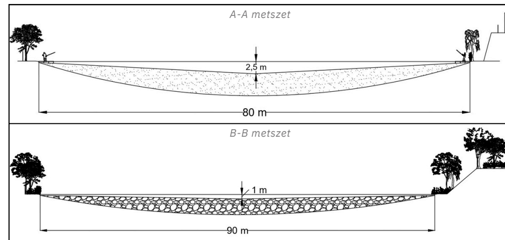
Felső- és Alsó-tó metszete (Saját ábra, AutoCAD)
