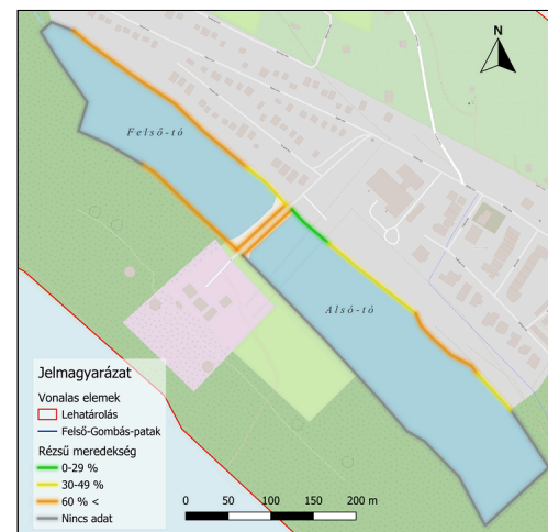
Rézsű meredekség és a területfelhasználás térképe (Saját ábra, QGIS)
